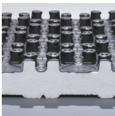
COSMO systémová deska UNI 30-2 s výstupky.
