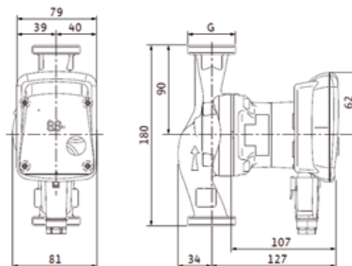
Rozměrový výkres
