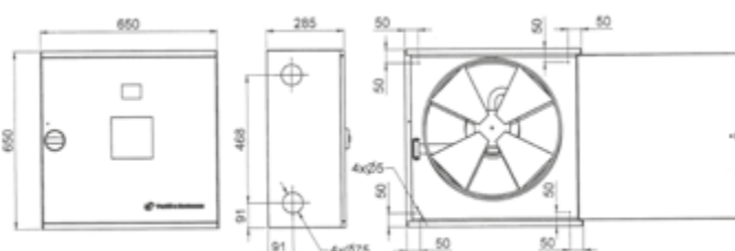
Hydrantový systém s tvarově stálou hadicí DN25
