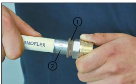
Detail správného zasunutí tvarovky COSMOFLEX.PRESS na trubku COSMOFLEX:
