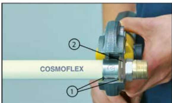
Správné založení vodícího plastového kroužku tvarovky do fixační drážky čelisti typu „B“
