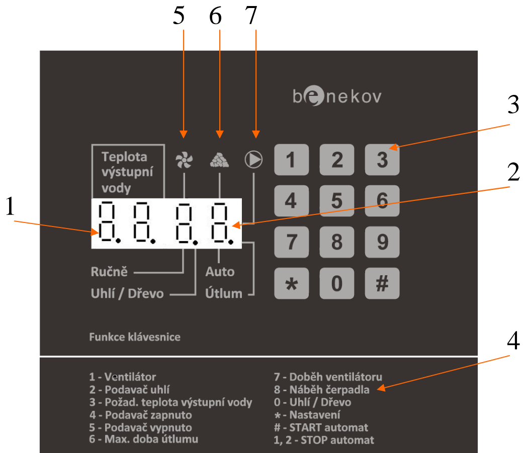
Obr. č. 1 Čelní panel regulátoru RKU1.5
