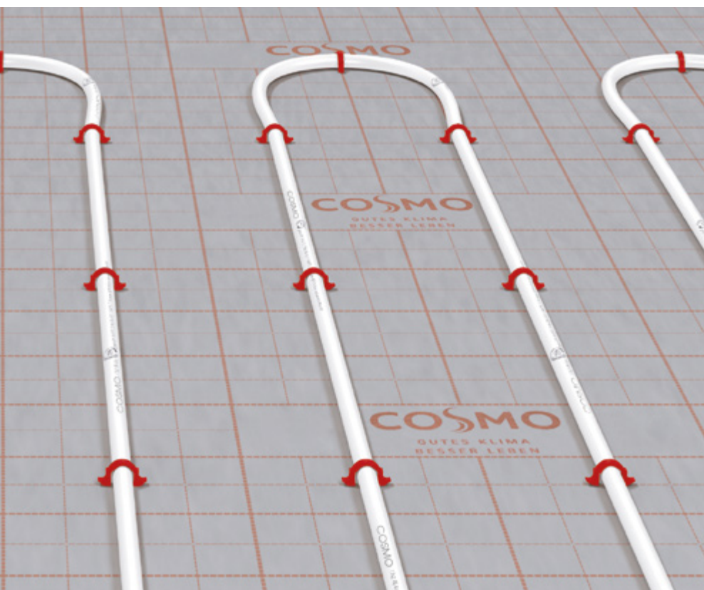
COSMO vícevrstvé potrubí s kyslíkovou bariérou PE-RT/AL/PE 16x 2mm DIN CERTCO 3V379MVR
