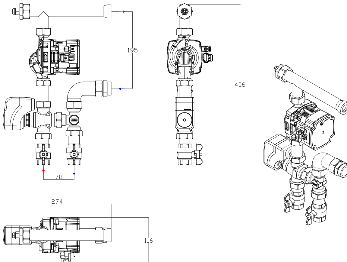
Rozměrové schéma:
