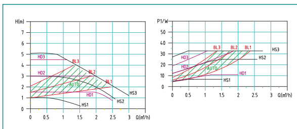
• TRICOE-5 III výkonová křivka
