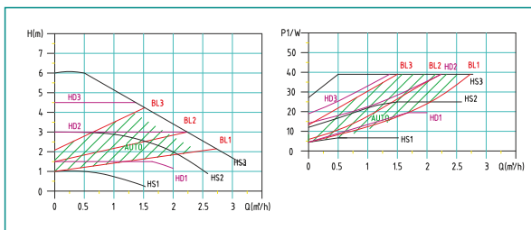
• TRICOE-6 III výkonová křivka
