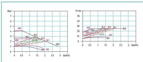
• TRICOE-4 III výkonová křivka
